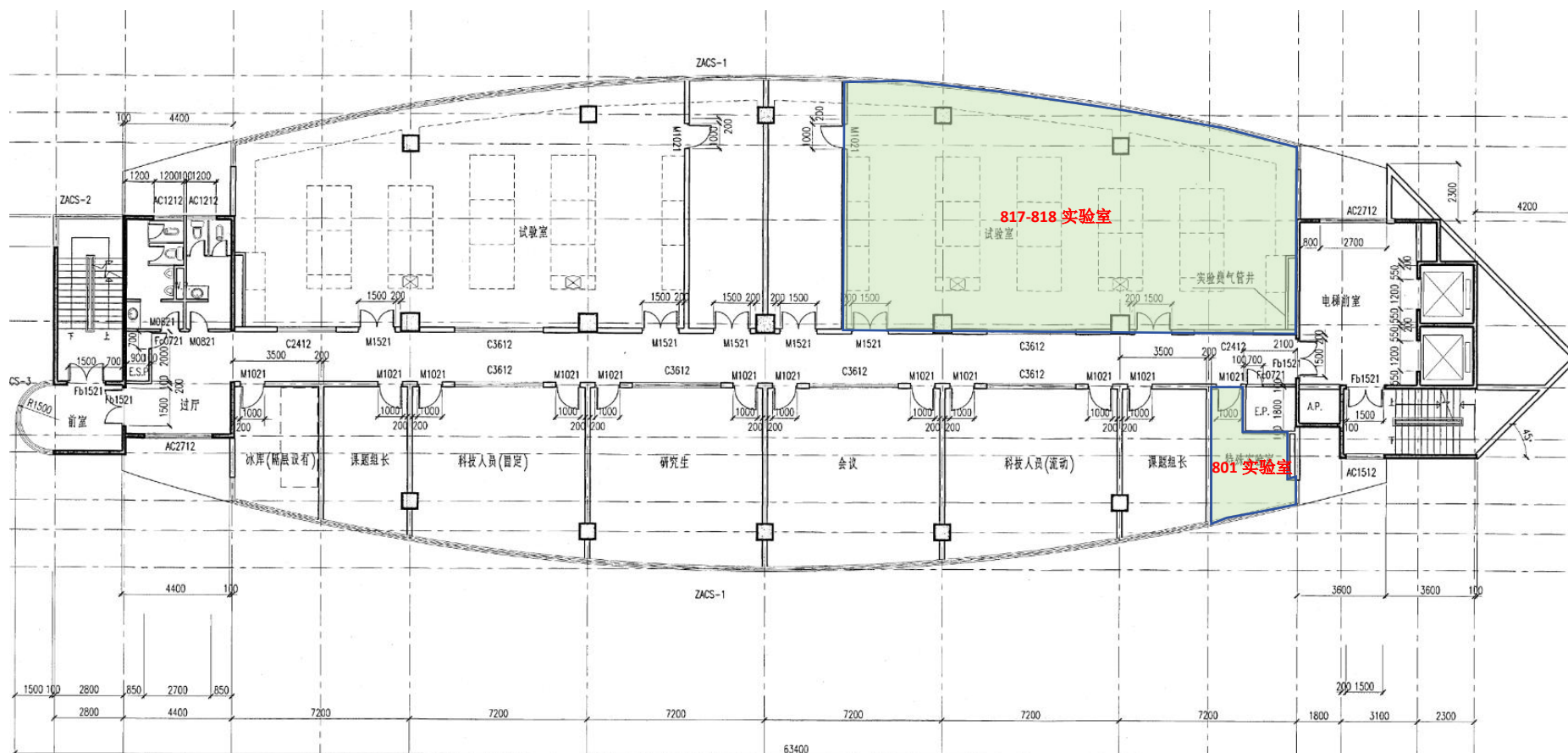
1 号楼 8 楼平面图
